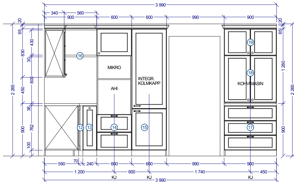
SEINAVADE B SKAALA 1:20
